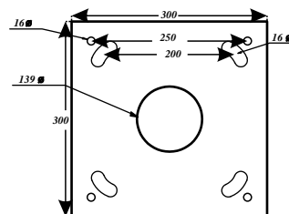
Platine d'ancrage
