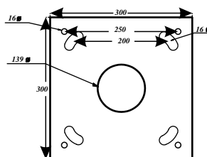
Platine d'ancrage
