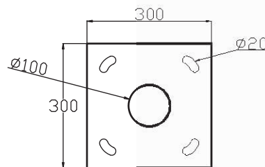
Platine d'ancrage
