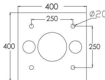
Platine d'ancrage
